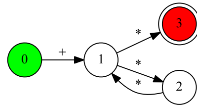
Рис. 2: Результат аппроксимации
