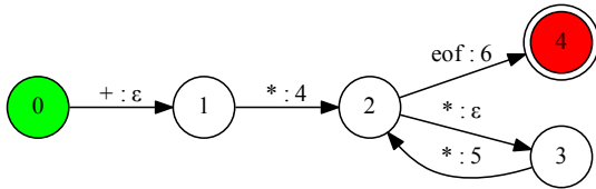
Рис. 5: Результат композиции
