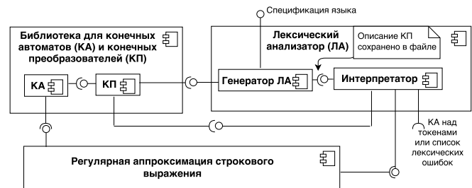
Рис. 7: Архитектура модуля для лексического анализа
