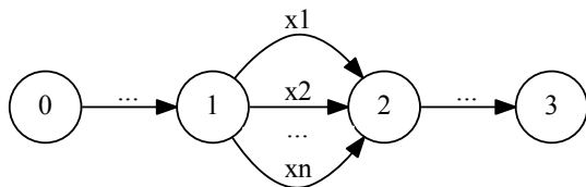
Рис. 12: Конечный автомат
