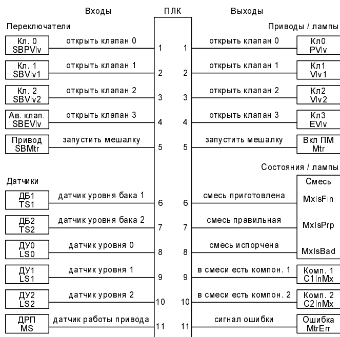
Рис. 2. Интерфейс установки для приготовления смесей
