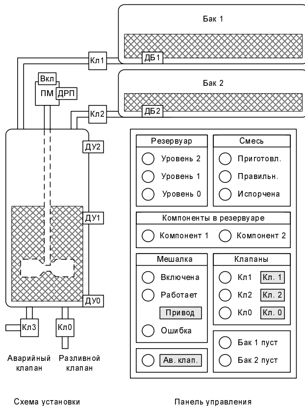
Рис. 1. Схема и панель управления установки для приготовления смесей
